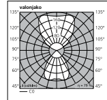
SYLWING S 3x28W
