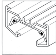
Kiskon korkeus 18 mm Kiskon leveys 30 mm
