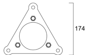
Asennusrauta betonivaluun
