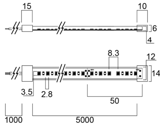
Flex Pro 48W CRI90 IP65
