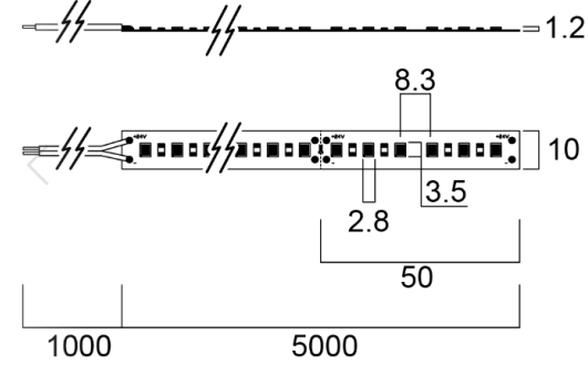
Flex Pro 48W CRI90 IP20
