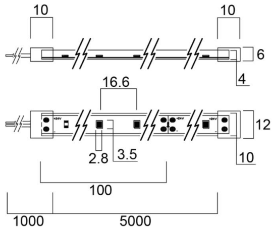
Flex Pro 24W CRI90 IP65
