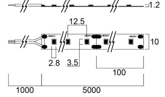
Flex Pro 72W CRI90 IP20
