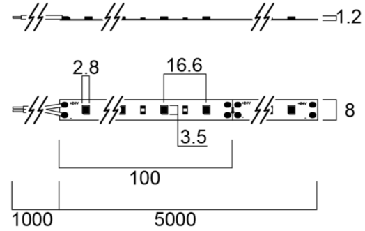
Flex Pro 24W CRI90 IP20
