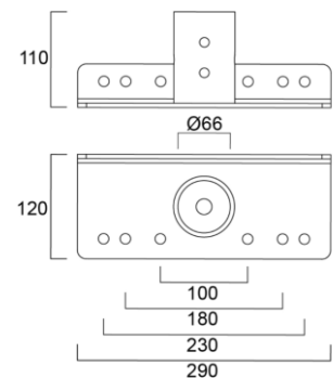
Pylväskiinnike pylvään päähän 60 mm
