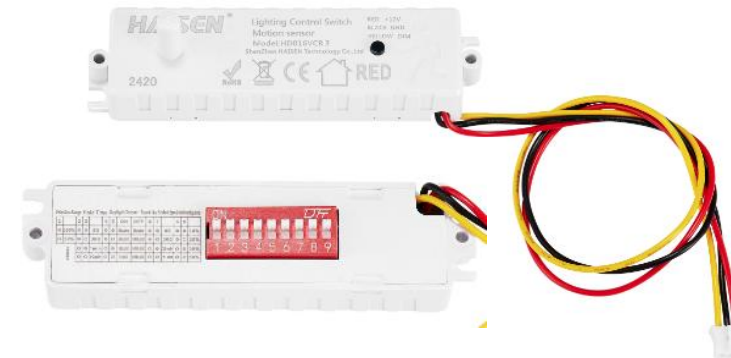
Liiketunnistinyksikkö 0040064
