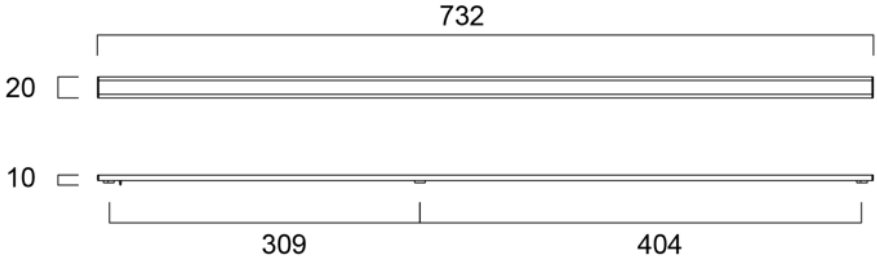
ylävalomoduuli
