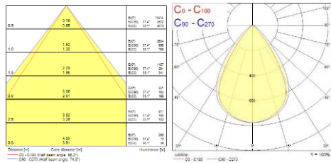
Mikroprisma
