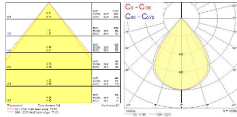
Valkoinen optiikka
