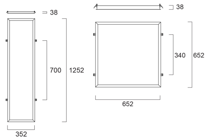
Asennuskehyykset kipsilevykattoon
