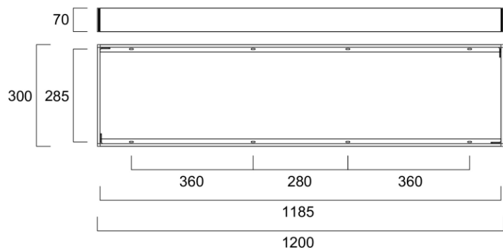
Pinta-asennuskehys 1200x300
