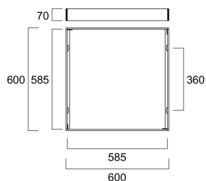
Pinta-asennuskehys 600x600
