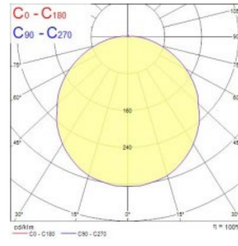
17W 3000K
