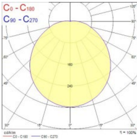
9W 3000K
