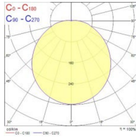
9W 4000K
