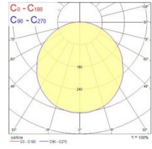
17W 4000K
