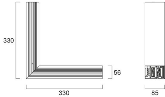
Valaistu L-kulma, pinta-/ripustusasennus
