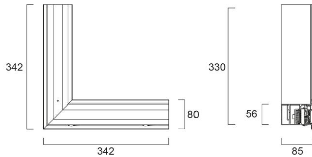
Valaistu L-kulma, uppoasennus
